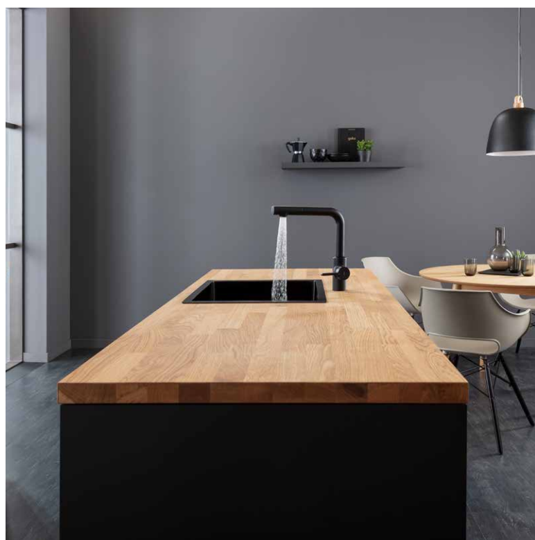
FIT Einhebel-Küchenarmatur L-Auslauf, schwenkbar, ausziehbare Brause, Ausladung 210 mm, Höhe 290 mm
