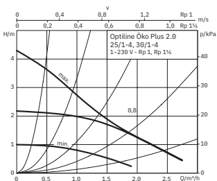
Kennlinien 4 Meter
