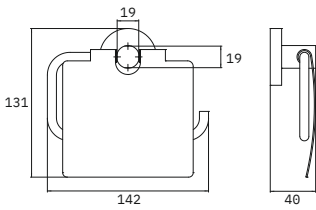
Papierhalter mit Deckel Art.-Nr. 30 830 56 000 000
