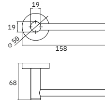
Papierhalter ohne Deckel Art.-Nr. 30 830 57 000 000
