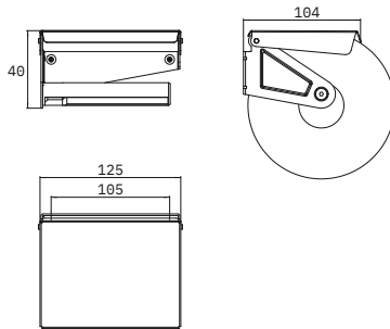
Papierhalter mit Deckel und Rolle Art.-Nr. 30 830 56 000 100
