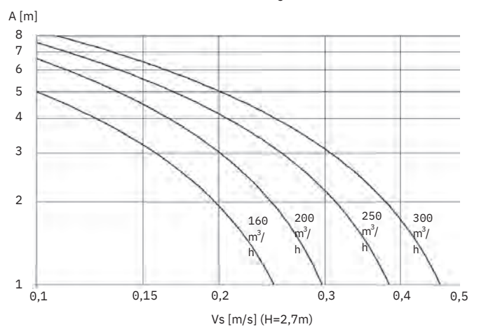
Maximale Strahlgeschwindigkeit V_s
