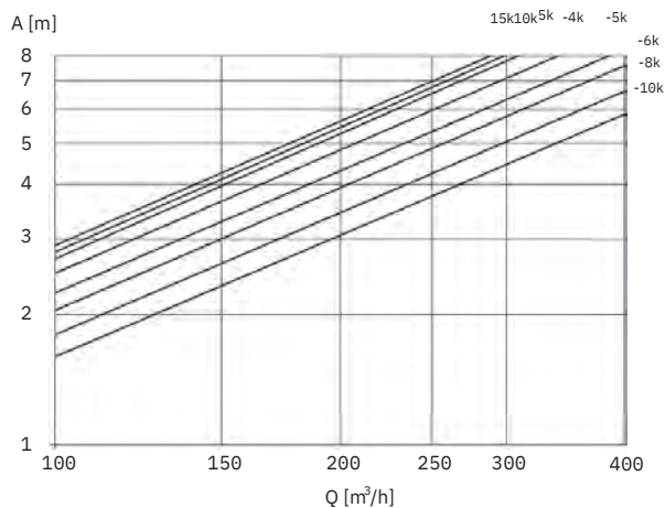
Abstand zwischen Drallausslässen Heizfall/Kühlfall
