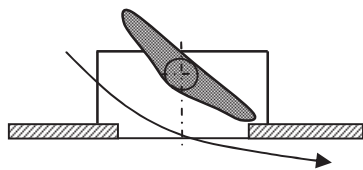
Lamellenstellung A
