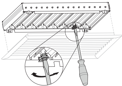
Die Einregulierung kann auch im eingebauten Zustand erfolgen
