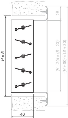
Anbauteil gegenläufige Mengenregulierung
