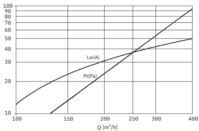
DV 300 Zuluft Druckverlust, Schallleistungspegel
