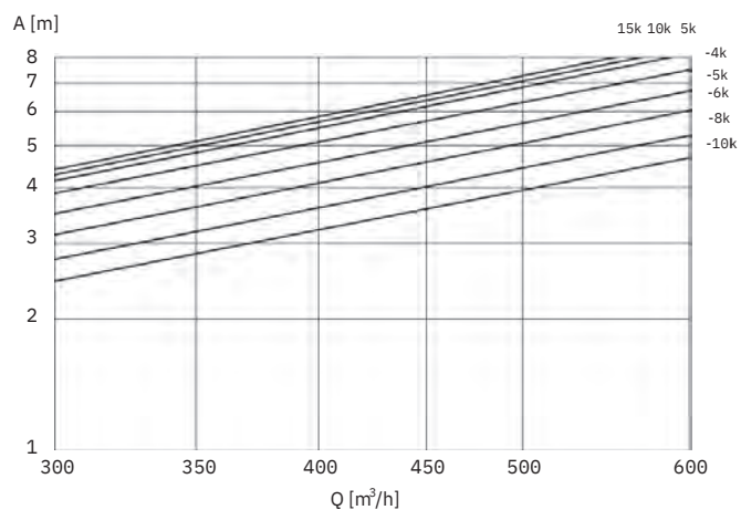
Abstand zwischen Drallausslässen Heizfall/Kühlfall
