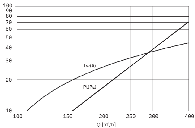
DV 400 Zuluft Druckverlust, Schallleistungspegel
