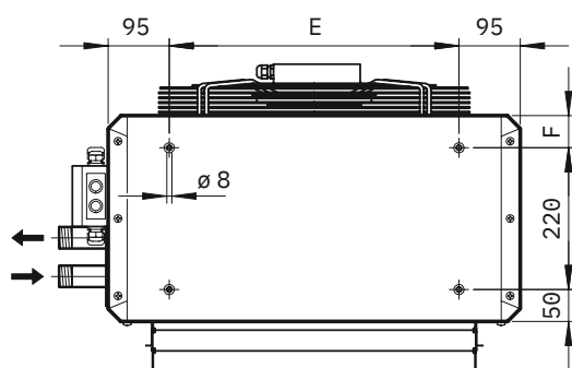
Draufsicht
