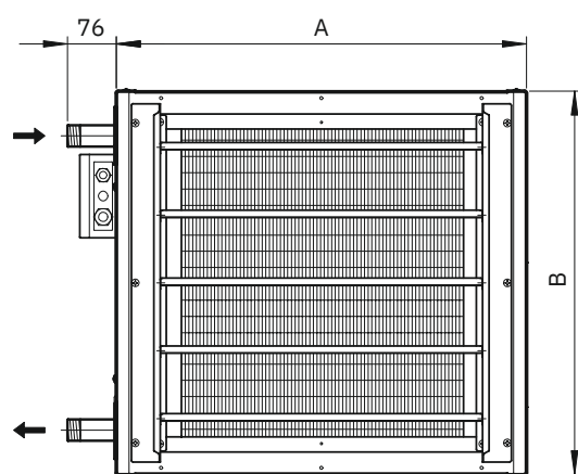
Vorderansicht
