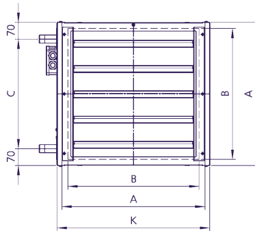
Vorderansicht
