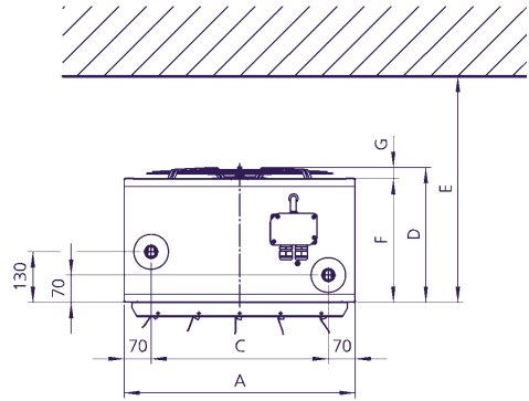
Deckenmontage
