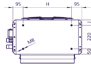
Befestigungsbohrungen
